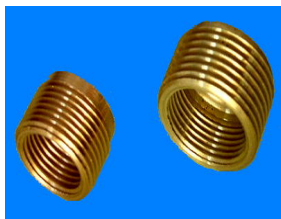
ERD
